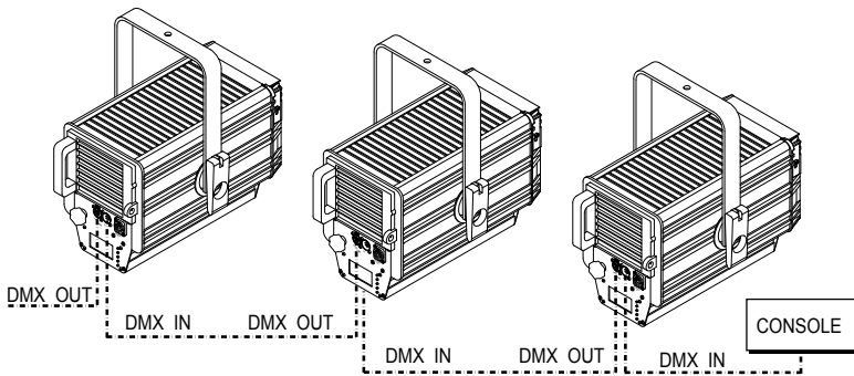
Fig. 4 Installazione MASTER/SLAVE - MASTER/SLAVE configuration
